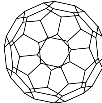
Fulereo
