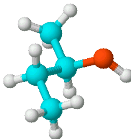
Estrutura 3D – modo bolas e varas
